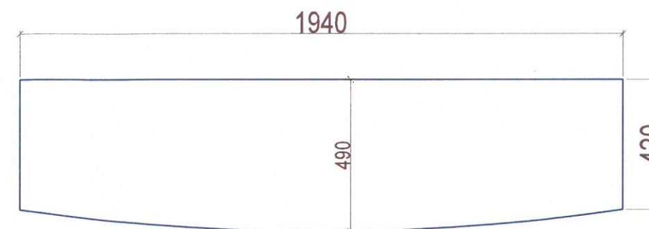
TOP VIEW CREDENZA TOP
